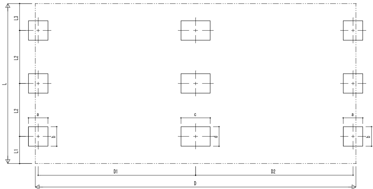
■基礎配置図
